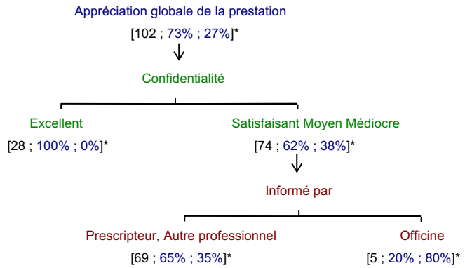
Figure 2 : Arbre de segmentation de l'appréciation de la prestation
