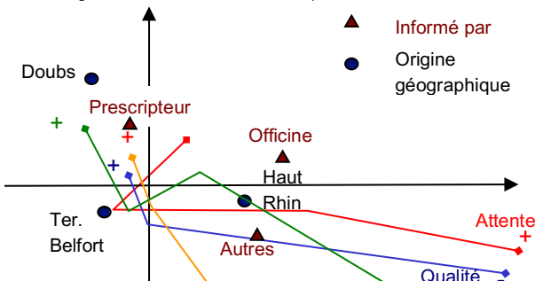
Figure 1 : AFCM Satisfaction des patients externes
