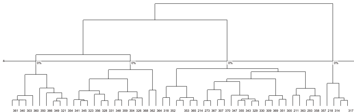
Classification hiérarchique directe (sur facteurs)
